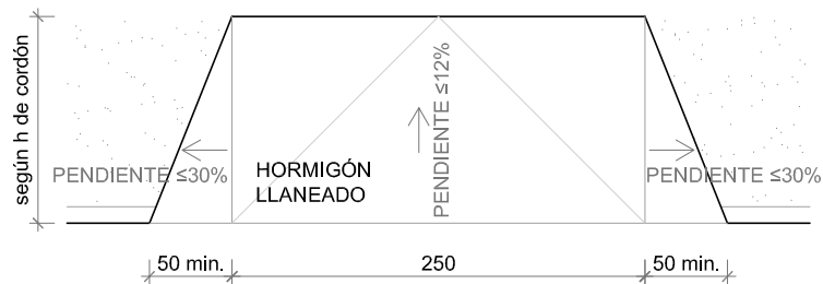
A. Planta
